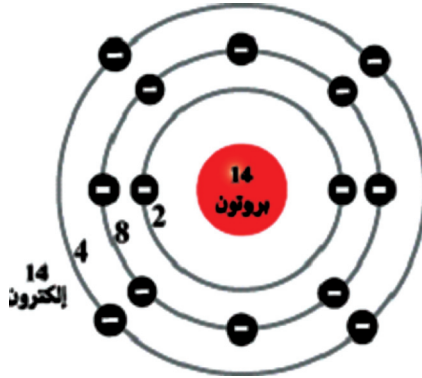
البناء الذري للسيليكون
